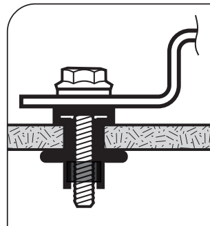
La Fig. 3.7 . Quand le boulon est serré, le corps en néoprène de l'écrou-douille est comprimé et dilaté à la fois, le forçant à se loger bien dans les filets du boulon et contre la surface interne du matériau de toit mince du VR.
